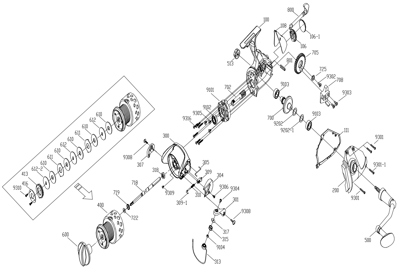
EZ - 90 Spare Parts
